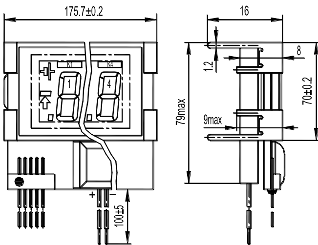
Рис.5 - ИВУ KF159Txx[2,4,7,9]-Dx, остальное - см. рис.1
