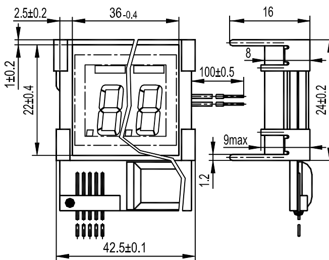
Рис.3 - ИВУ KF128Tx1xx[1-4]-Dx, остальное - см. рис.1
