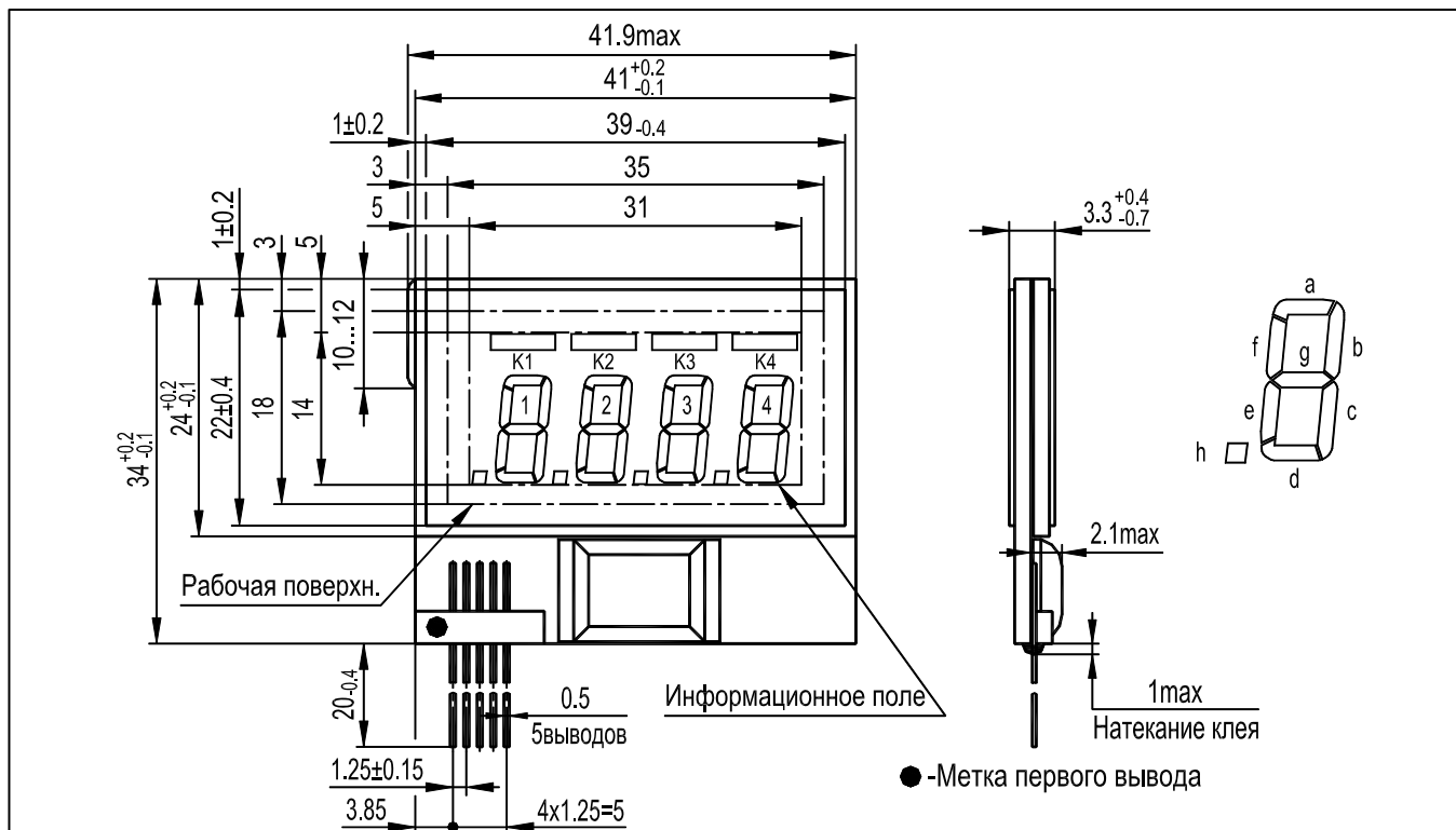
Рис.1 - ИВУ CF128Tx1xx[1-4]
