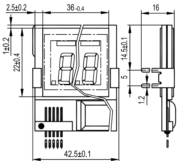
Рис.2 - ИВУ KF128Tx1xx[1-4], остальное - см. рис.1
