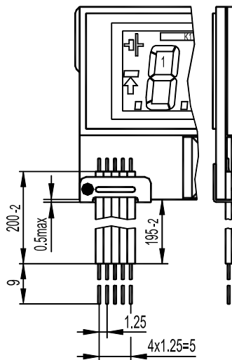
Рис.2 - ИВУ CS152Tx2xx[2,4,7,9], остальное - см. рис.1
