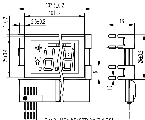
Рис.3 - ИВУ KF152Tx2xx[2,4,7,9], остальное - см. рис.1
